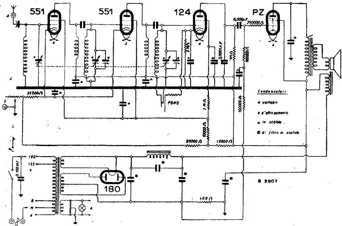
RADIOMARELLI - MOD. « CORIBANTE »
