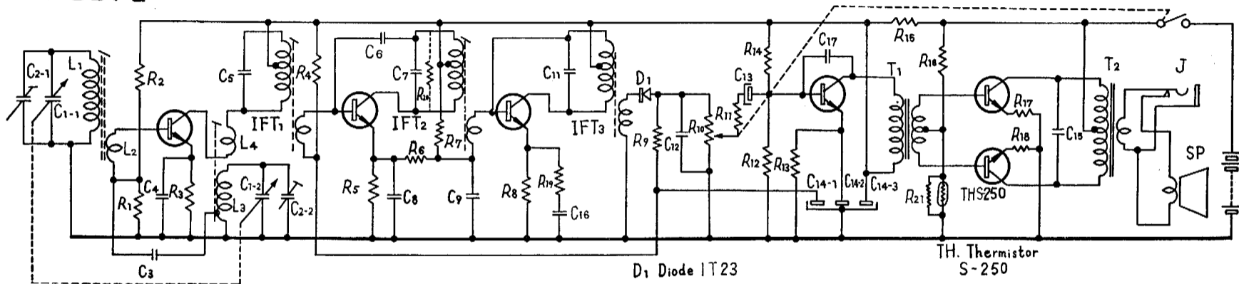
Fig. 13.4. - Schema di tascabile a 6 transistor NPN e 1 diodo Sony.
